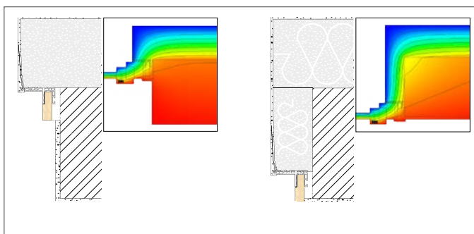
TERMOGRAFIE DI C1 SUPER FILO E CENTRO MURO
